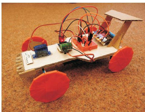
Autíčko na dálkové ovládání micro:bitem
